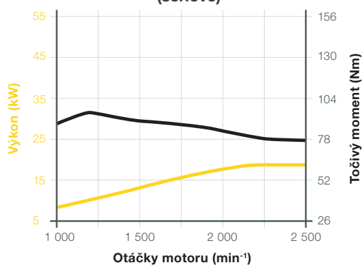
Výkonnostní křivka Yanmar 3TNV82A-B; 18,5 kW; stupeň V (sériově)
